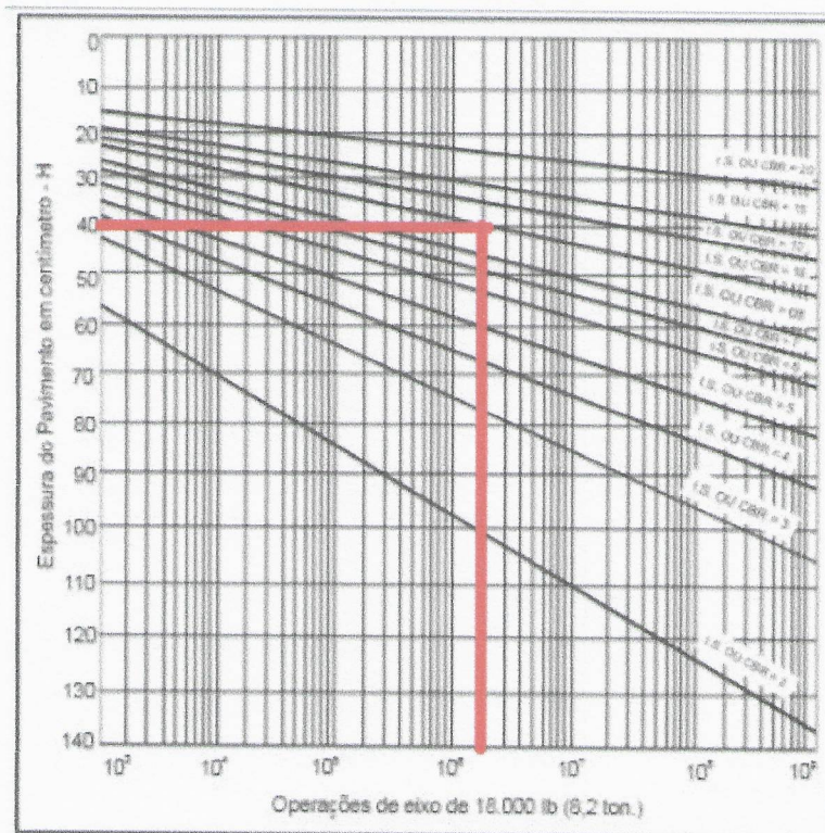
FIGURA 01: Ábaco de dimensionamento
