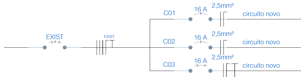
ESQUEMA UNIFILAR – QUADRO GERAL – ADICIONAR CIRCUITOS
