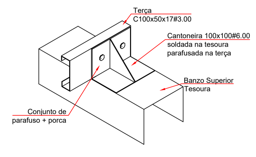
Detalhe Fixação das Terças Esc: 1/10
