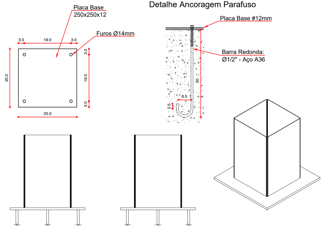
DETALHE FIXAÇÃO DOS PILARES METÁLICOS NA SAPATA Sem Escala
