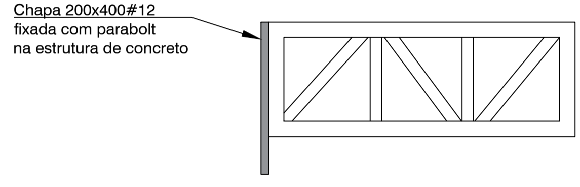
Ligação Tesoura com Pilar de Concreto Existente Esc: 1/10
