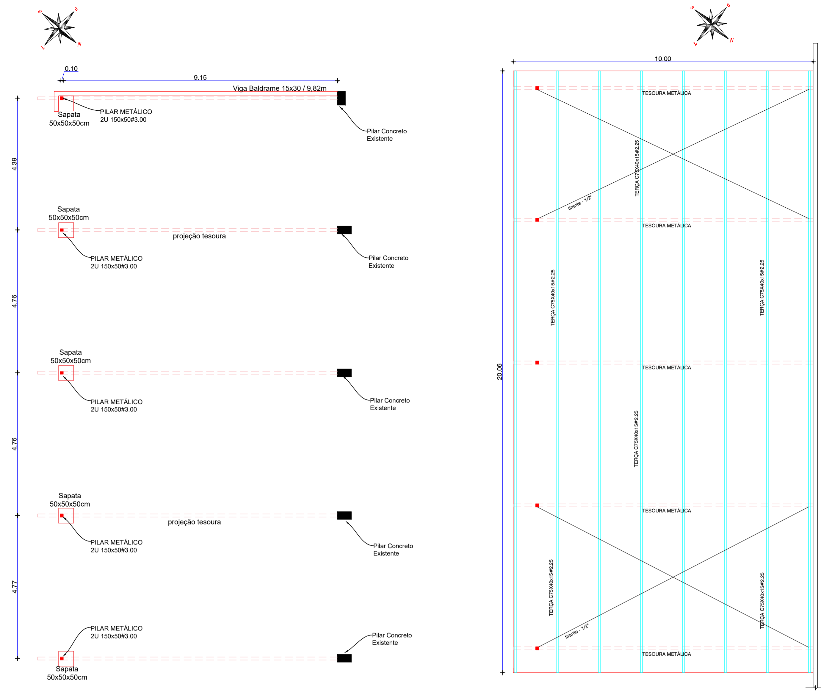
PLANTA DE COBERTURA Escala: 1/75
