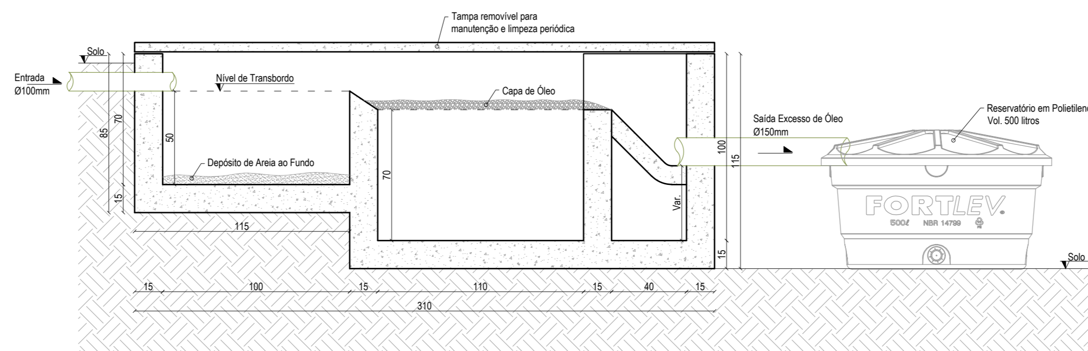
CORTE AA Caixa de Separação do Efluente Escala: 1/20
