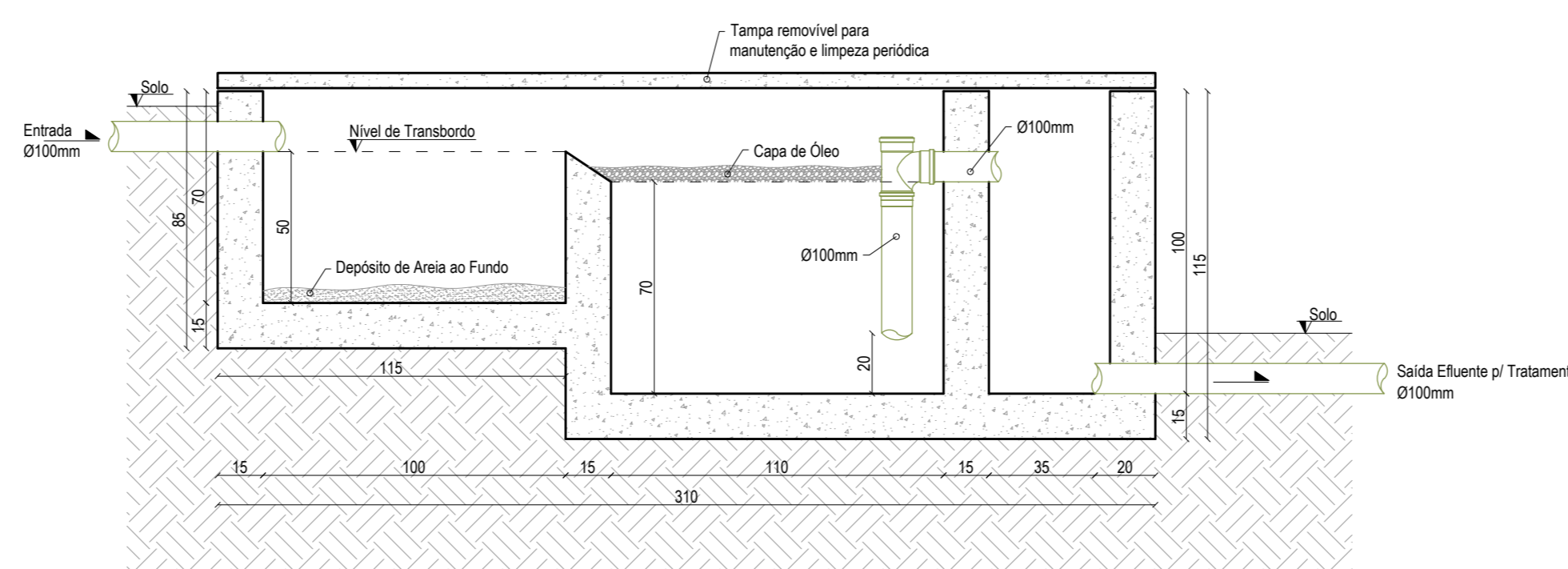
CORTE BB Caixa de Separação do Efluente Escala: 1/20
