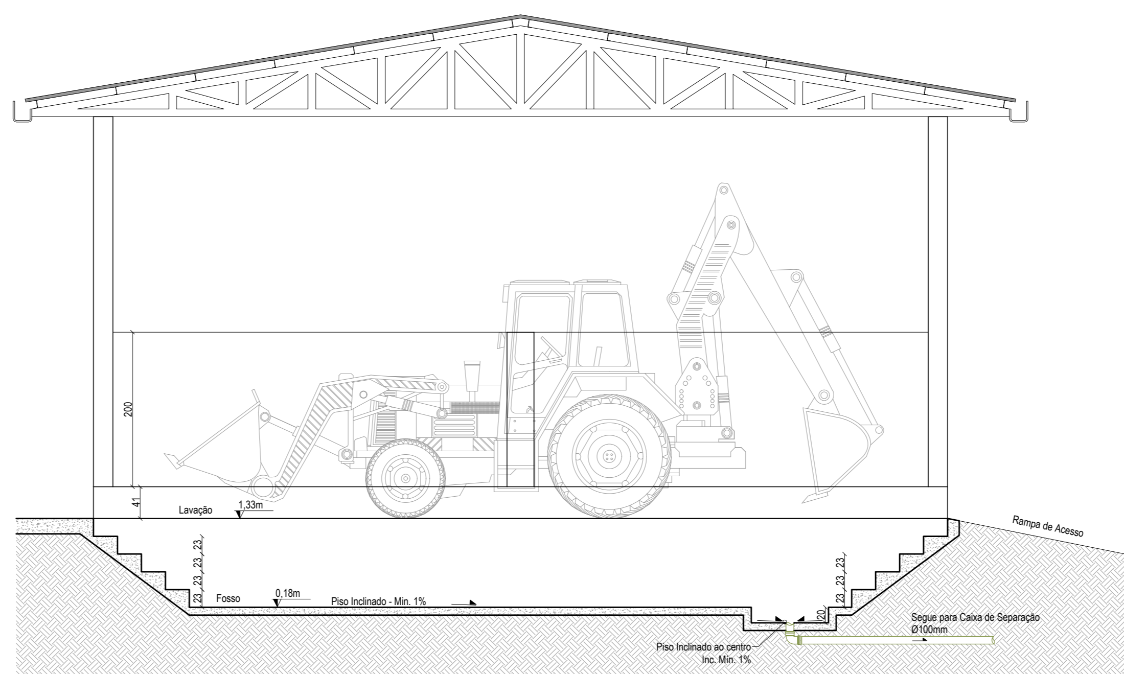
CORTE Fosso Escala: 1/50
