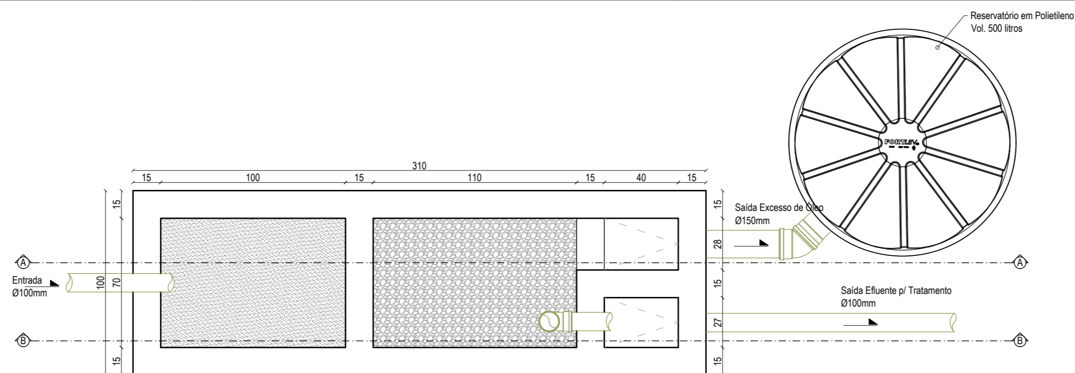
PLANTA BAIXA Caixa de Separação do Efluente Escala: 1/20
