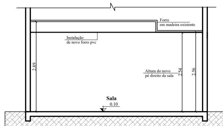
Corte A-A
