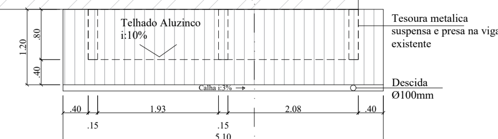
Planta Baixa Cobertura Frontal Esc.: 1/75
