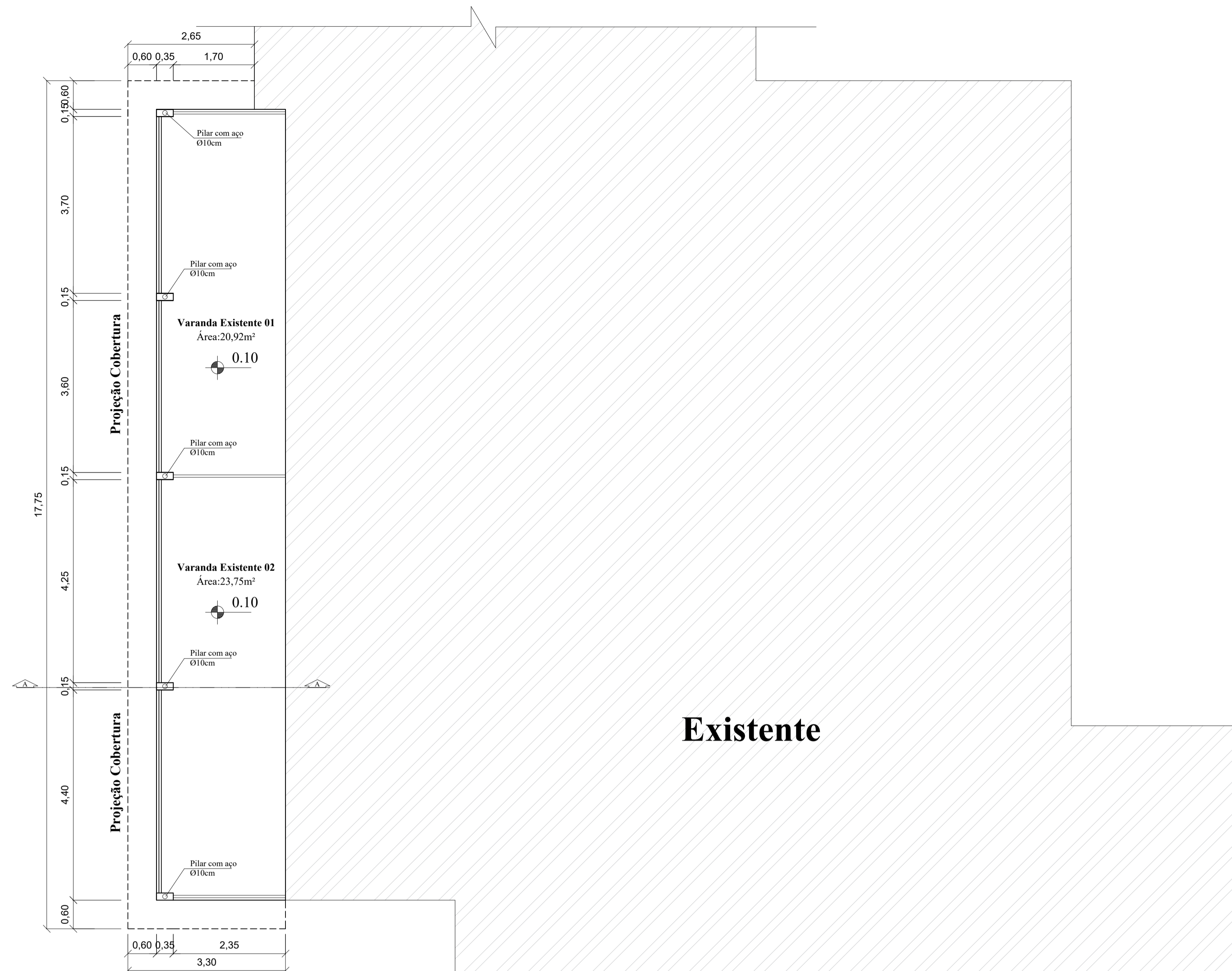
Planta Baixa Toldo A: 40,53m 2 Esc.: 1/75
