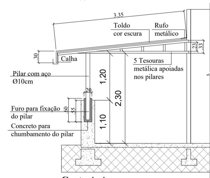
Corte A-A Esc.: 1/75
