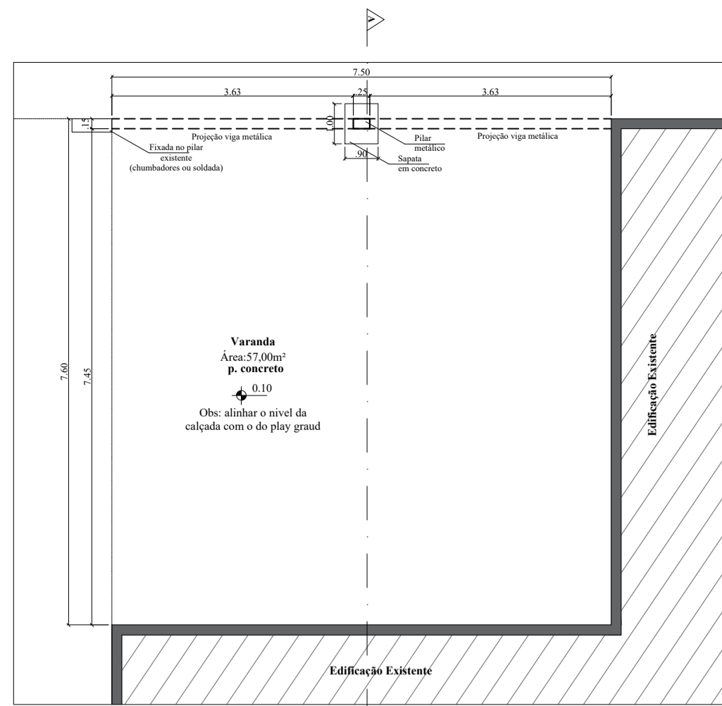
Planta Baixa Cobertura Área: 57,00 m 2 Esc.: 1/75
