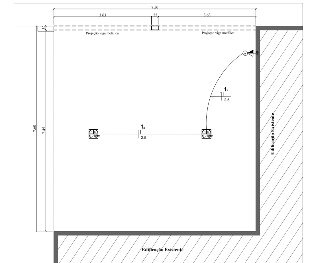
Planta Baixa Cobertura Elétrica Esc.: 1/75
