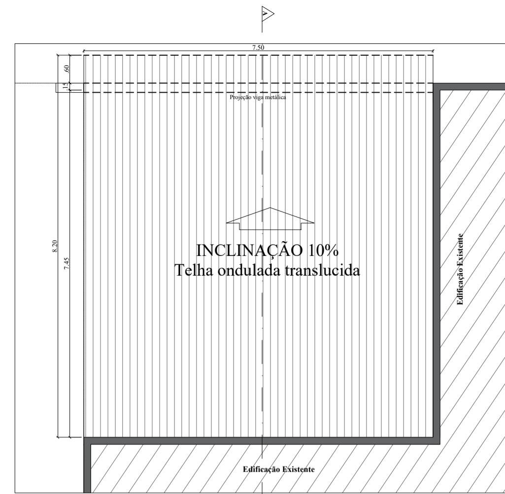
Planta de Cobertura Área: 57,00 m 2 Esc.: 1/75
