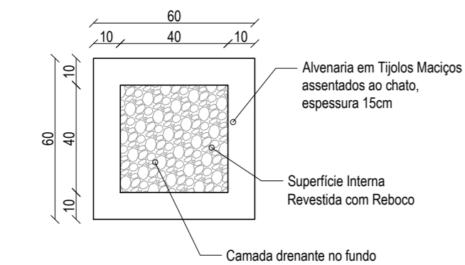
PLANTA BAIXA Caixa de Passagem Interna Escala: 1/20
