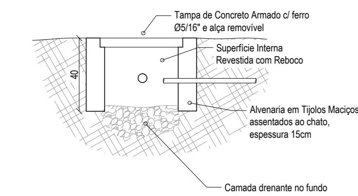
CORTE Caixa de Passagem Interna Escala: 1/20
