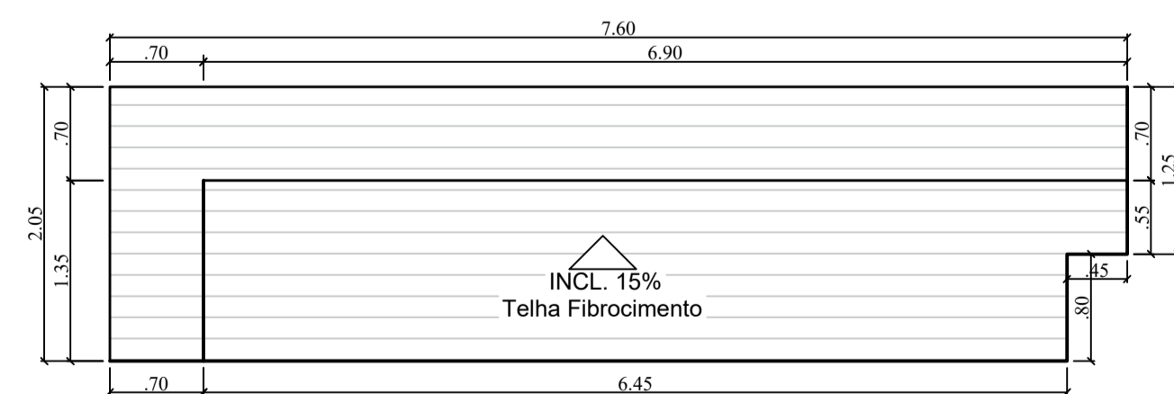
Cobertura Metálica Esc 1:50
