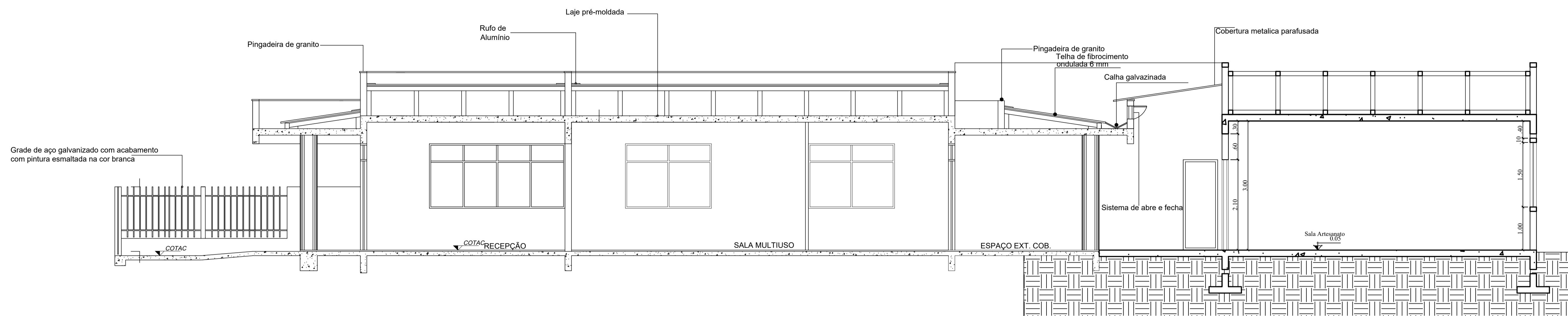
Corte B-B Esc 1:50
